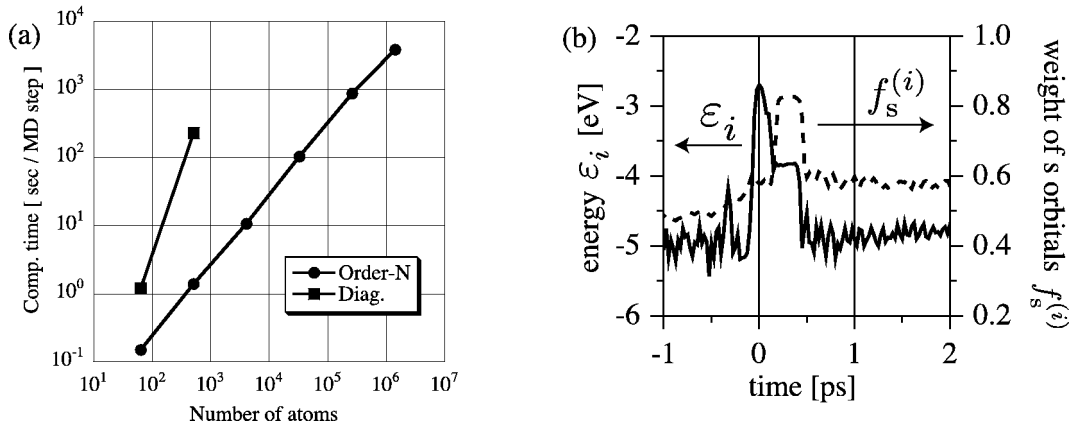
図 1: (a) 摂動オーダー N 法 (Order-N) と厳密対角化法 (Diag.) における、計算時間のシステムサイズ (原子数) 依存性 (第 1 章図 1.1)。標準的のワークステーションを用いて計算された。(b) 破壊素過程における、ワニア状態の観測。エネルギー \epsilon_i = \langle \phi_i | \hat{H} | \phi_i \rangle と s 波成分の重み f_s^{(i)} を示した (第 7 章 2 節図 7.5)。
