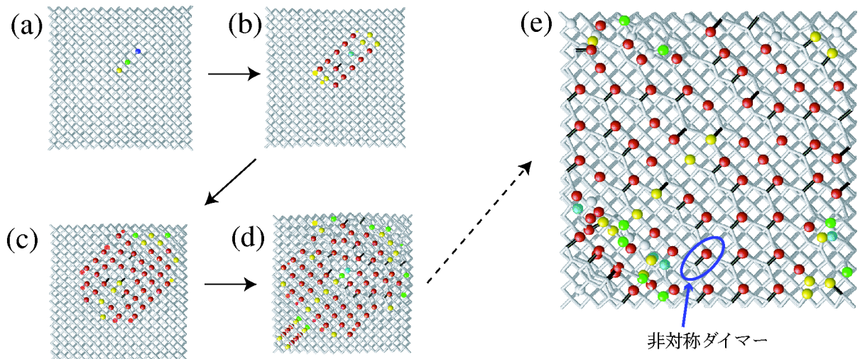
図 2: 4501 原子からなるナノ結晶シリコンの破壊過程。初期構造に含まれる欠陥ボンドを起点として、非対称ダイマーを含んだ亀裂 (001) 面が生成される。ワニア状態を、結合軌道 (ロッド) または原子軌道 (球) として描いた。後者は、 f_s^{(i)} によって色分けされている。また、黒い結合は、表面再構成によって形成された結合を表す (第 7 章 5 節図 7.21 よりの抜粋)。
