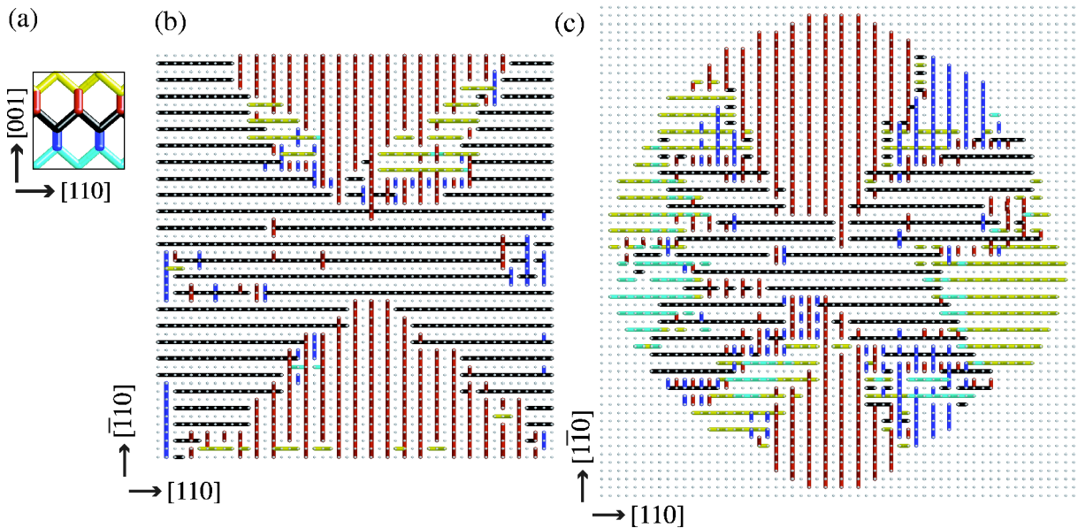
図 3: 亀裂 (001) 面におけるステップ構造のサンプルサイズ依存性。(a) 色分けの例: 理想結晶構造におけるボンドサイトの、原子層による分類。(b)(c) 結合が切れたボンドサイトを、理想結晶構造において図示している。(b) 約 3 万原子系、(c) 約 12 万原子系。(b) ではサンプル全体の断面を、(c) では中央付近のみの断面を描画している。サンプルサイズは、 [110] または [\bar{1}\bar{1}0] 方向に、(b) が約 10nm、(c) が約 20nm。(第 7 章 6 節図 7.29, 図 7.34)。
